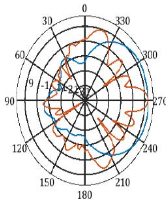
f=2700MHz, Co@2-cuts
